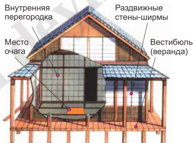
Традиционный японский дом. Схема
